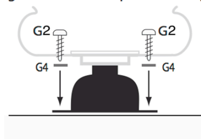
Trageschiene/Gummipuffer befestigen
